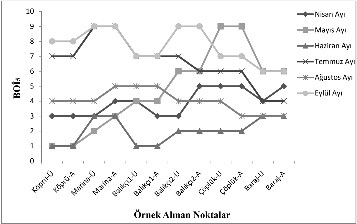
Şekil 5. Borçka Baraj Gölünde BOI 5 aylara göre değişimi
