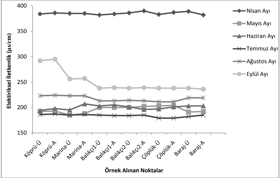
Şekil 4 . Borçka Baraj Gölünde elektriksel iletkenliğin ( \mu\text{S}/\text{cm} ) aylara göre
