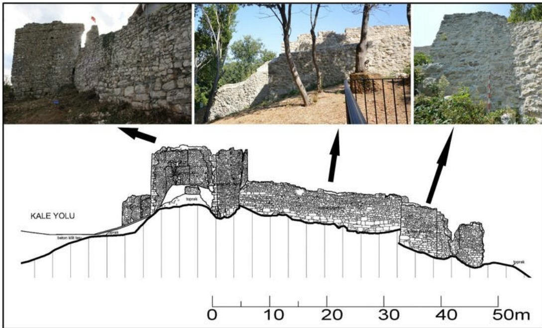
Görsel 7: Doğu Sur Cephe Çizimi ve Detay Görünüşleri (Konuralp Müzesi Arşivi ve E. Verim)
