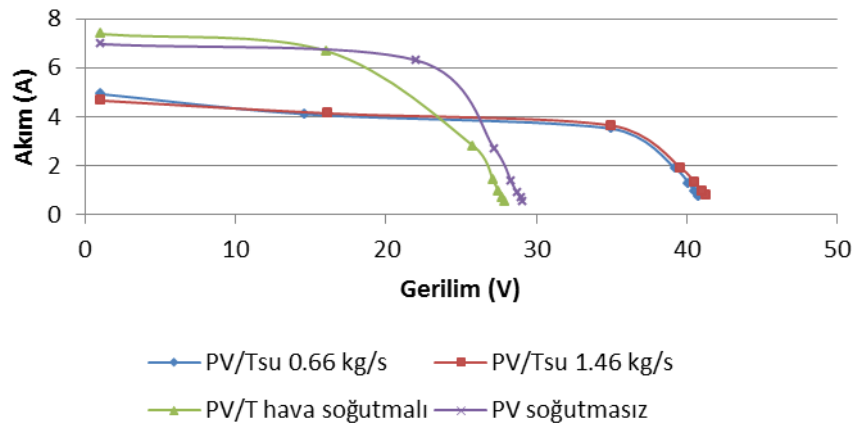
Şekil 11. Akım – Gerilim eğrisi (Panel Açılı: 33°, Güneş Işınım Değerleri ort. 900 W/m 2 )
