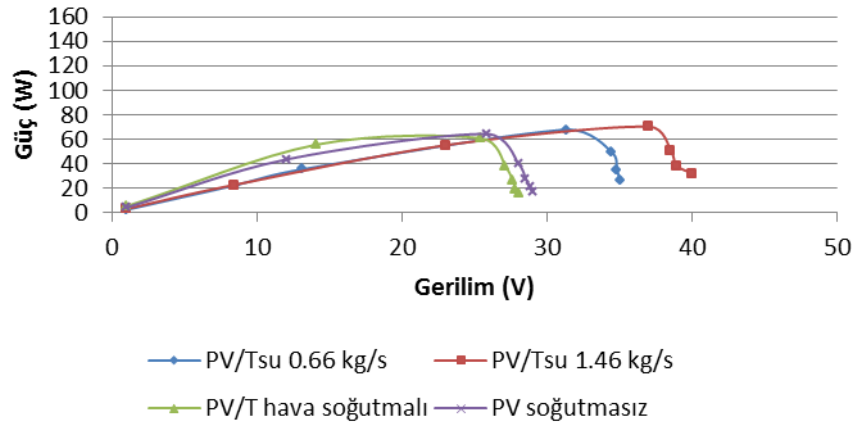
Şekil 10. Güç – Gerilim eğrisi (Panel Açılı: 33°, Güneş Işınım Değerleri ort. 600 W/m 2 )
