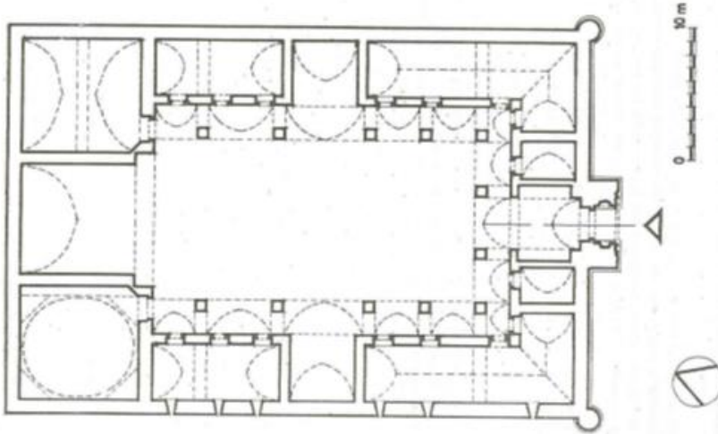
Şekil 16. Kayseri Sahibiye Medresesi, Plan, (Sözen, 1970)
