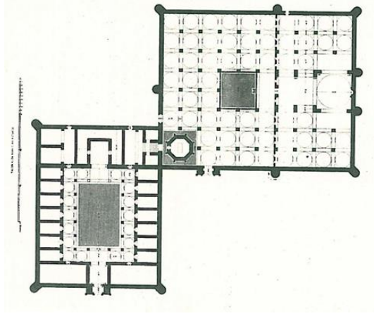
Şekil 9. Huand Hatun Camii ve Medresesi, Plan (Texier, 1849)
