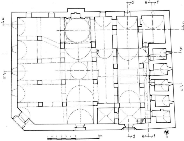
Şekil 2. Kılık Camii ve Medresesi Plan ( Yurdakul, 1974)
