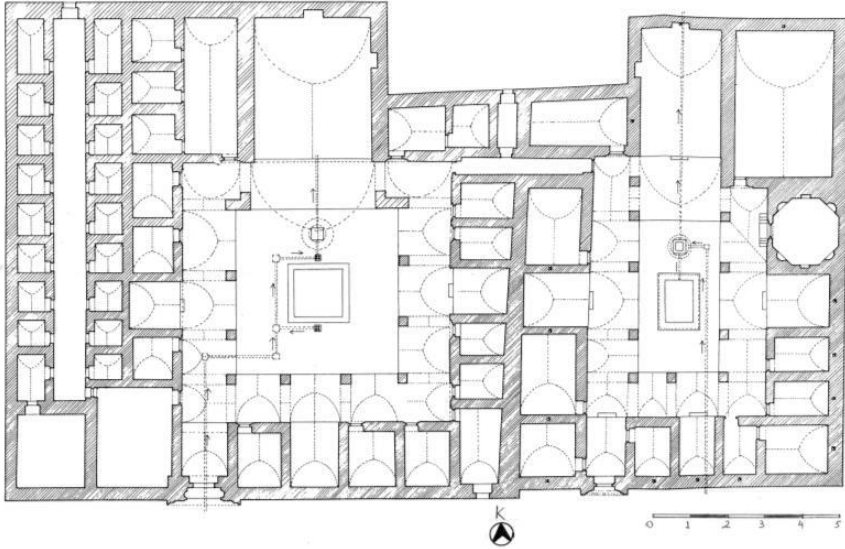
Şekil 5. Kayseri Çifte Medrese, Plan (VGM Arşivi)
