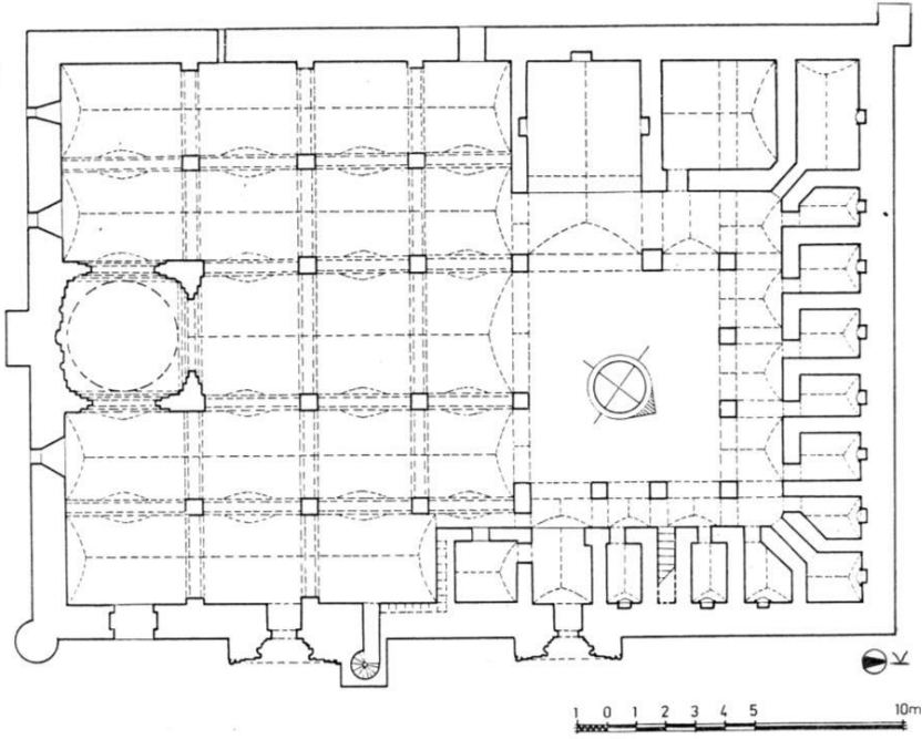
Şekil 14. Kayseri Hacı Kılıç Camisi ve Medresesi, Plan (Öney, 1966)
