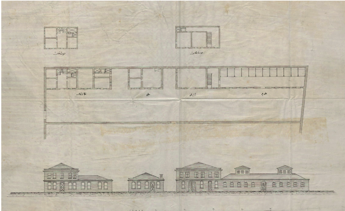
Resim 1: Sadrazam Hayreddin Paşa Konağı, BOA, Plan, Proje, Kroki, (PLK.p), 1373.
