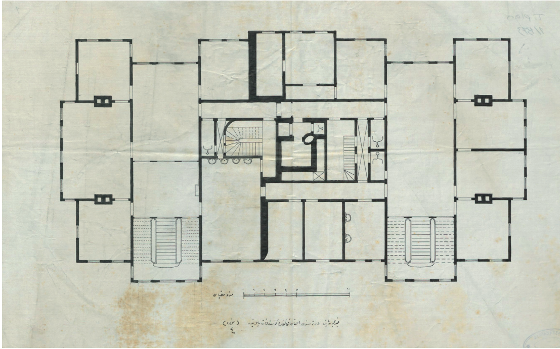
Resim 3: Sadrazam Hayreddin Paşa Konağı'nın üst kat planı, BOA, PLK.p., 1373.
