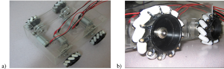
Şekil 1. Swedish mekanizmalı mobil robotun; a) Üstten görünümü, b) Yandan görünümü
