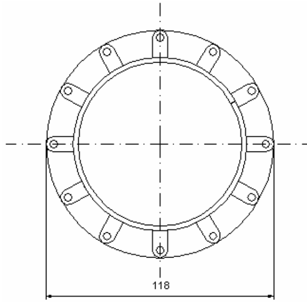
Şekil 11. Swedish mekanizmalı tekerleğin soldan görünüş teknik resmi
