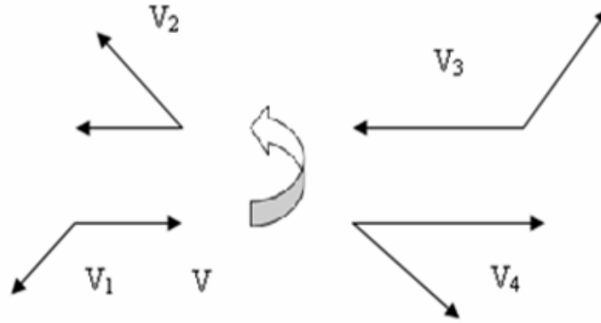
Şekil 5. Swedish mekanizmalı mobil robotun düşey eksen etrafında dönme hareketinin hız vektörleri
