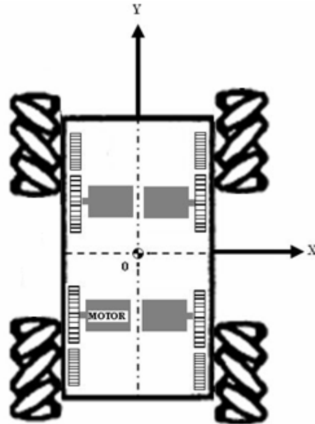
Şekil 7. Silindirik ruloların her teker üzerinde yerleştirme pozisyonları
