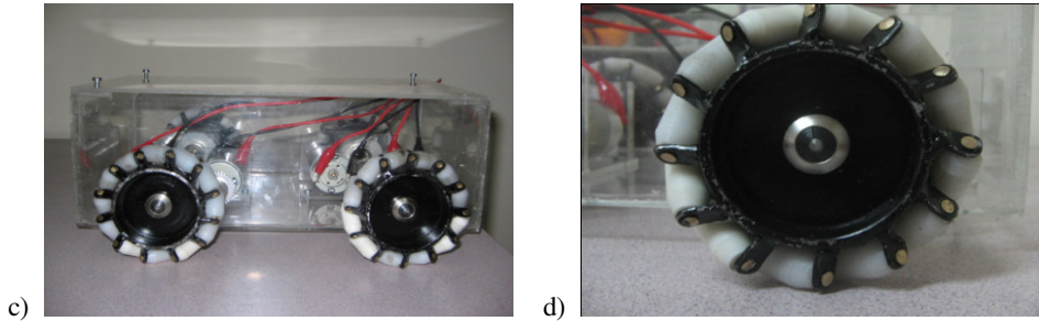
Şekil 2. Swedish mekanizmalı mobil robotun; c) Soldan görünümü, d) Bir tekerinin görünümü
