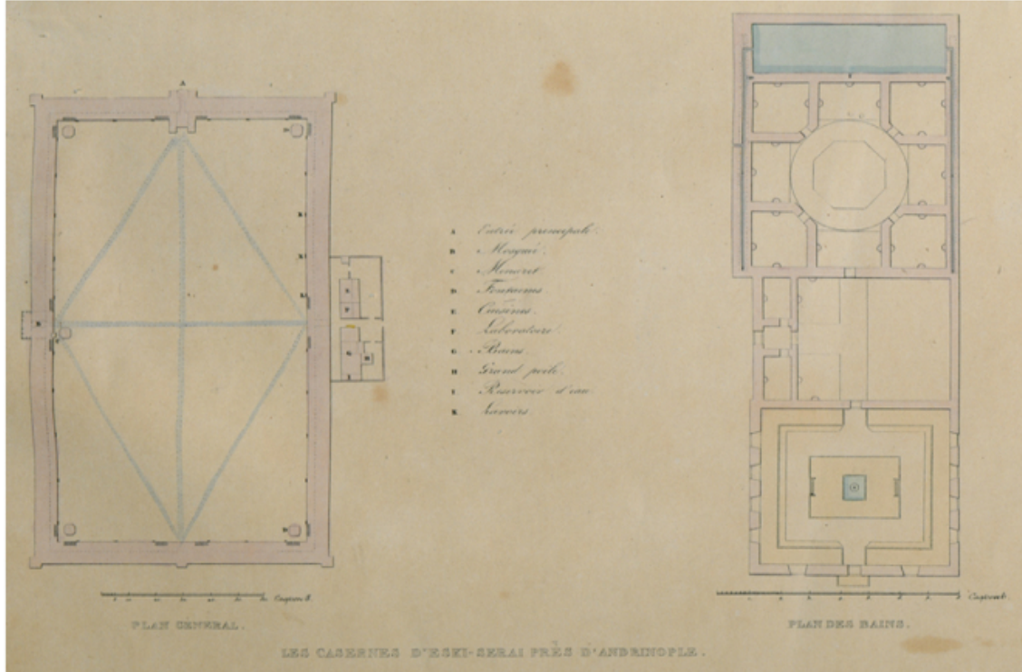
Şekil 2. 1829-1830 Yıllarına ait Edirne Piyâde Kışla-i Hümâyûnu Çizimleri: a. Kışla ve Hamamın Vaziyet Planı; b. Hamam Planı
