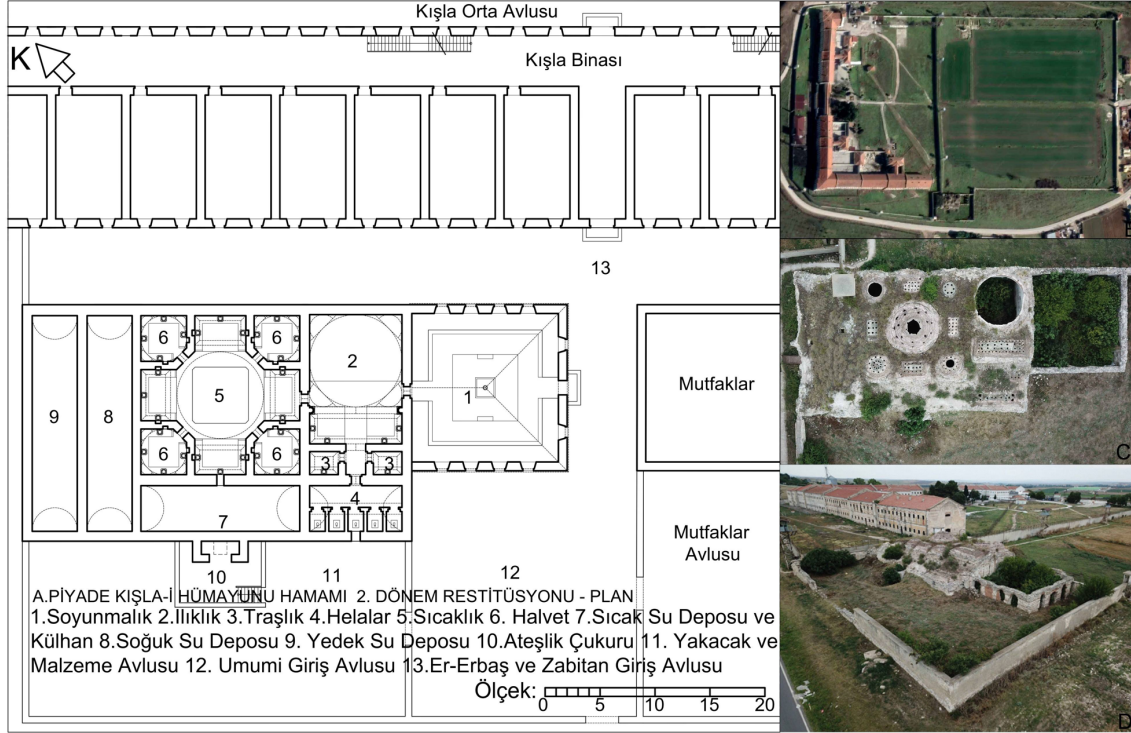
Şekil 17. A. Piyâde Kışla-i Hümayûnu Hamamı ve Çevresinin 2. Dönem Restitüsyonu-Plan; B. Piyâde Kışla-i Hümayûnu (Kapalı Cezaevi) ve Hamamı Hava Fotoğrafı, 2019; C. Hamamın Üst Örtüsünün Kuşbakışı Fotoğrafı, 2021; D. Güneybatı ve Güneydoğu Cephesi, 2021
