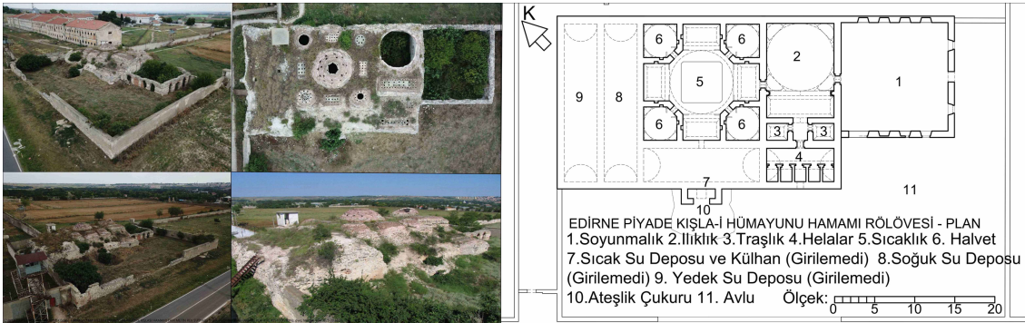
Şekil 7. Piyâde Kışla-i Hümayûnu Hamamı Güneydoğu, Güneybatı ve Kuzeybatı Cephelerini Gösterir Hava Fotoğrafları ile Mevcut Durum Planı
