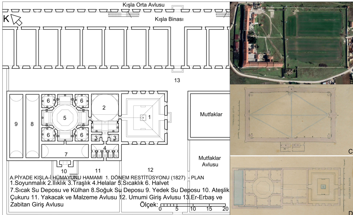
Şekil 16. A. Piyâde Kışla-i Hümayûnu Hamamı ve Çevresinin Sultan II. Mahmud Devri'ne ait 1. Dönem Restitüsyonu (1827) – Plan; B. Piyâde Kışla-i Hümayûnu (Kapalı Cezaevi) ve Hamamı Hava Fotoğrafı, 2019; C. 1829-1830 Yıllarında Kışla ve Hamamın Vaziyet Planı; D. 1829-1830 Yıllarında Hamamın Planı
