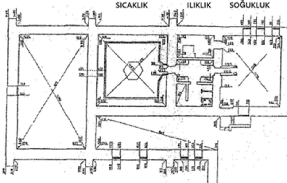
Şekil 4. Davud Paşa Kışlası Hamamı Planı
