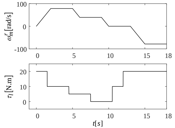
Şekil 3. Sürücü sistemine verilen hız referansı ve motora uygulanan yük momentini değişimleri
