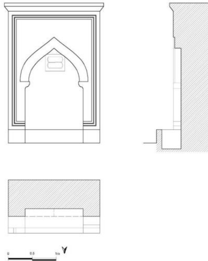
Çizim 2. Belören Köyü Çeşmesi Cephe, Kesit ve Plan Çizimi (Çerkez'den)
