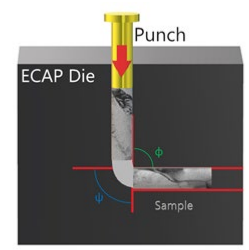
Figure 1. Angles in the ECAP pattern (EKAP kalbındaki açılar)
