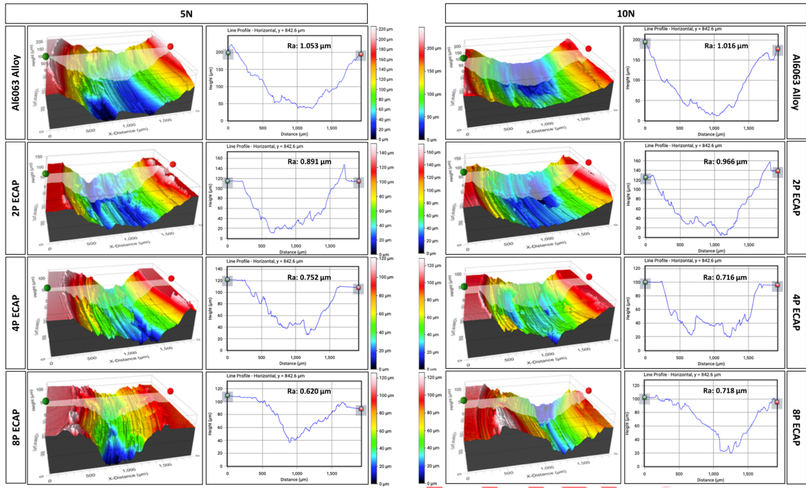
Figure 10. 3D profilometer analyses of Al6063 alloy samples with 2, 4 and 8 pass ECAP treatment under 5 and 10N loads (5 ve 10N yük altında 2, 4 ve 8 geçişli ECAP işlemine tabi tutulan Al6063 alaşım numunelerinin 3B profilometre analizleri)
