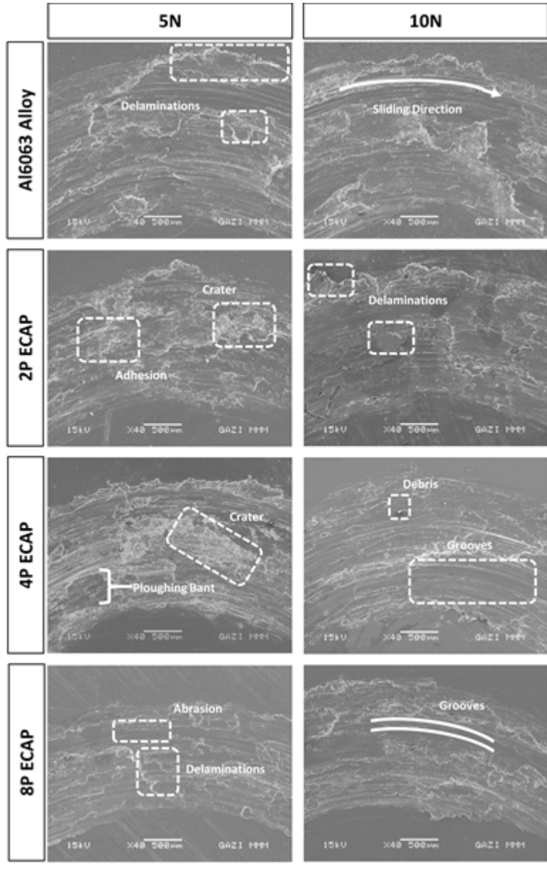
Figure 9. SEM analysis of 5 and 10N worn surfaces of Al6063 alloy, 2, 4 and 8 pass ECAP treated samples (Al6063 alaşımlarının 5 ve 10N aşınmış yüzeylerinin SEM analizi, 2, 4 ve 8 geçişli ECAP ile işlenmiş numuneler)
