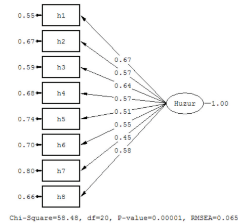
Şekil 1. Huzur Ölçeği'nin Yol Diyagramı ve Faktör Yükleri
