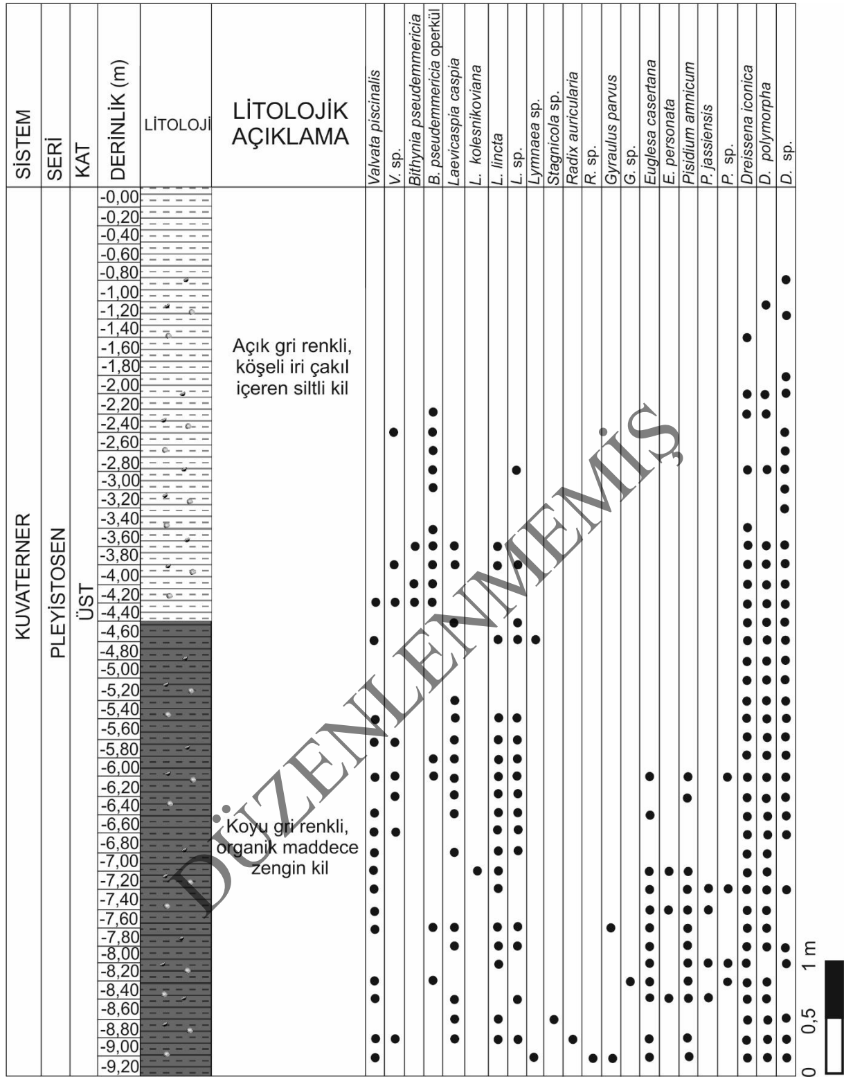
Şekil 4. Sk-1 Sondaj logu.
