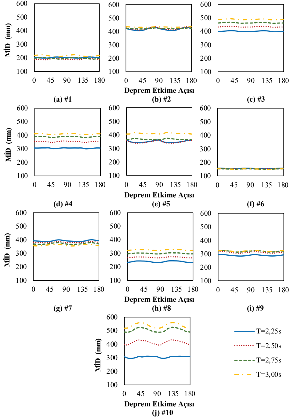
Şekil 8. Farklı etkiye açılara ve izolasyon periyoduna bağlı olarak yürütülen analizler sonucunda MCE deprem seviyesi için elde edilen MİD
