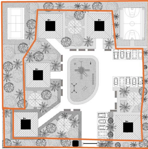
A- Gaziantep – Öğr.6: Vaziyet Planı Etüdü
