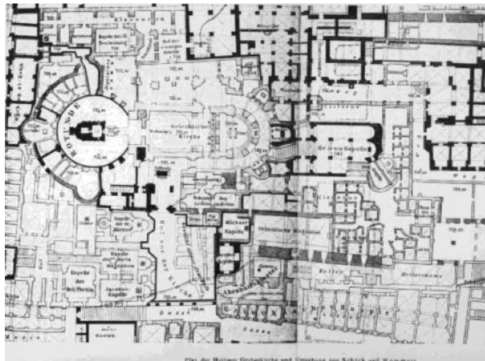
Şekil 11: Schick tarafından 1898'de hazırlanan Kutsal Kabir ve çevresinin planı, görüntü conradschick.wordpress.com'dan alınmıştır.
