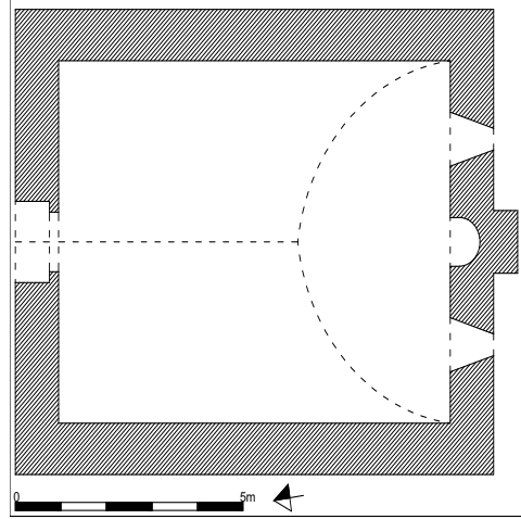
Şek. 15: Yılkent Mescidinin olası orijinal planı
