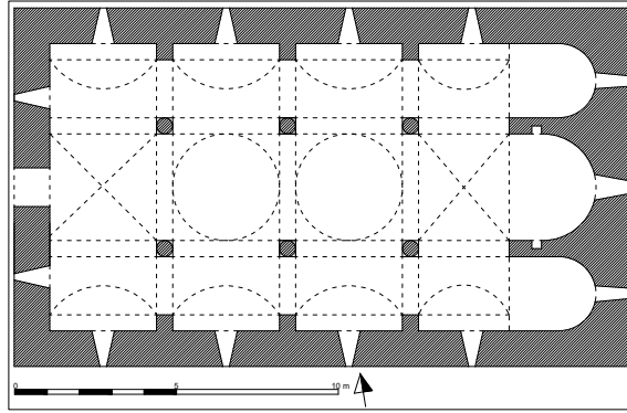
Şek. 14: Mescidin kuzeyindeki kalıntının olası orijinal planı
