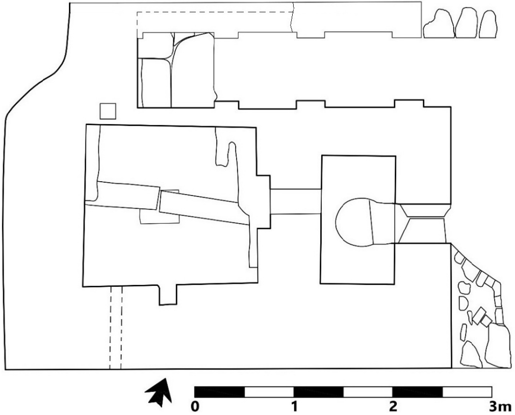
Şekil 3. Hamam sıcaklık seviyesindeki planı
