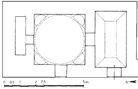
Şekil 5. Bolu'daki konak hamamının planı (Öztürk 1997)
