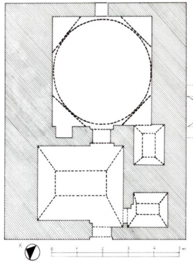
Şekil 8. Kayseri Tavlusun Bektaşoğlu Konağı Hamamı'nın planı (Aslan 2012)
