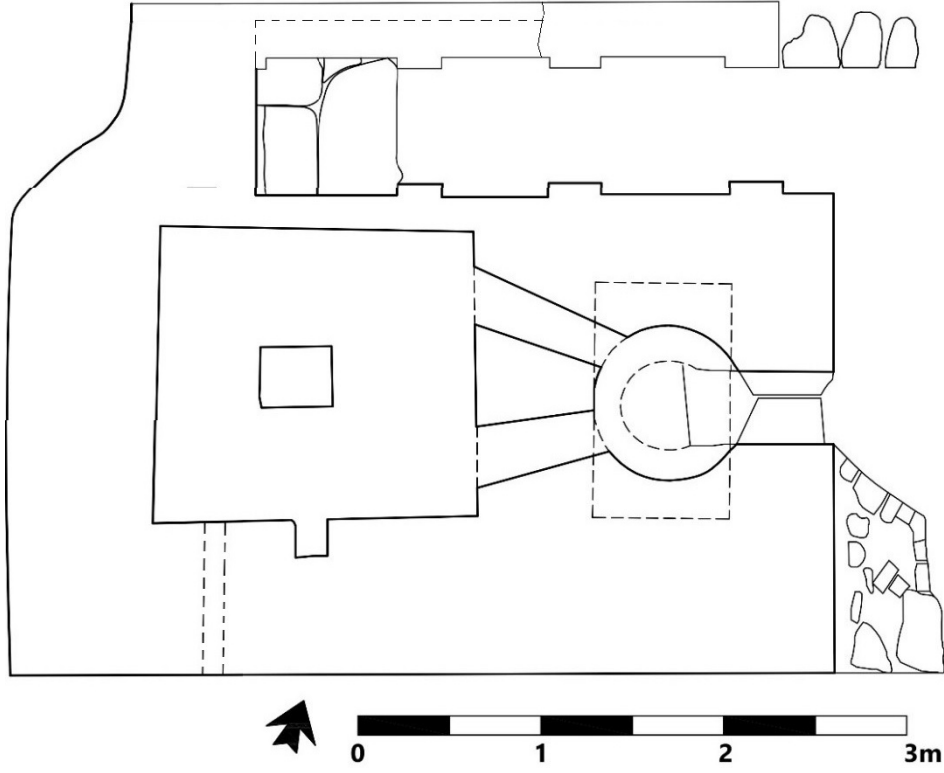
Şekil 4. Hamamın cehennemlik ve ocak seviyesindeki planı
