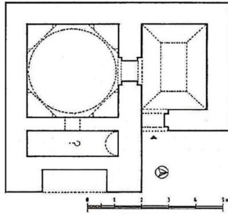
Şekil 7. Yozgat Lök Köyü Karaca Bey Konağı Hamamı planı (Kutlu 2022)
