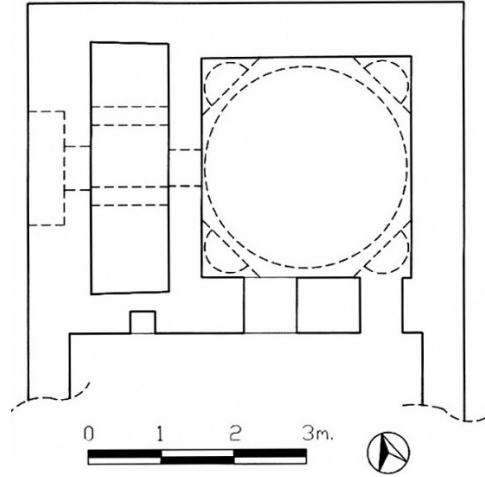
Şekil 6. Çanakkale Burhan Köyü Hamamı (Uysal 2014)
