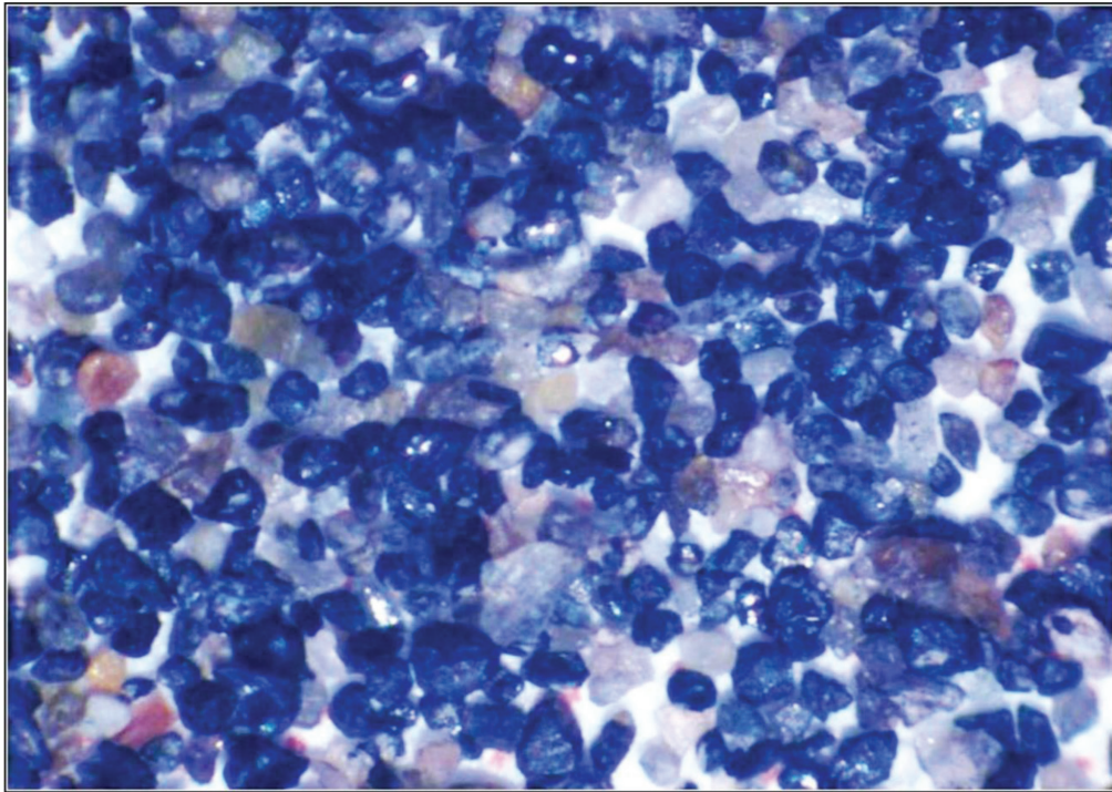
Şekil 7. Konsantrasyon plaser örneği içinde bulunan kromit ve diğer ağır minerallerin mikroskopik görünümü.
