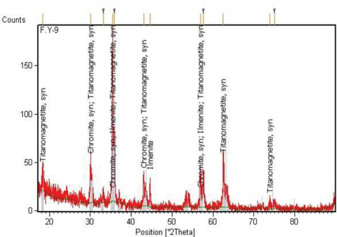
Şekil 8. Ağır mineral konsantrisi içinde bulunan minerallerin dağılımını gösteren XRD diyagramı Figure 8. The XRD diagram showing the distribution of minerals in heavy minerals concentration.
