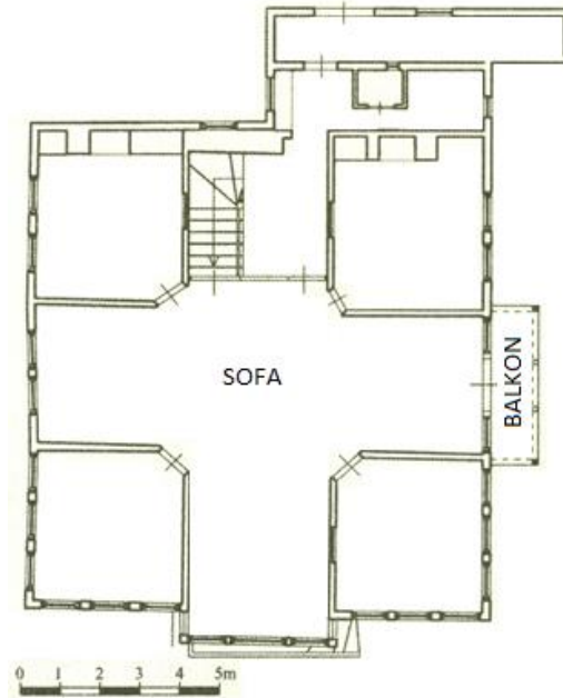
Şekil 11. Geleneksel Taraklı konut planına ait bir örnek; Taraklı Çakıroğlu Konağı 2.Kat planı [9].
