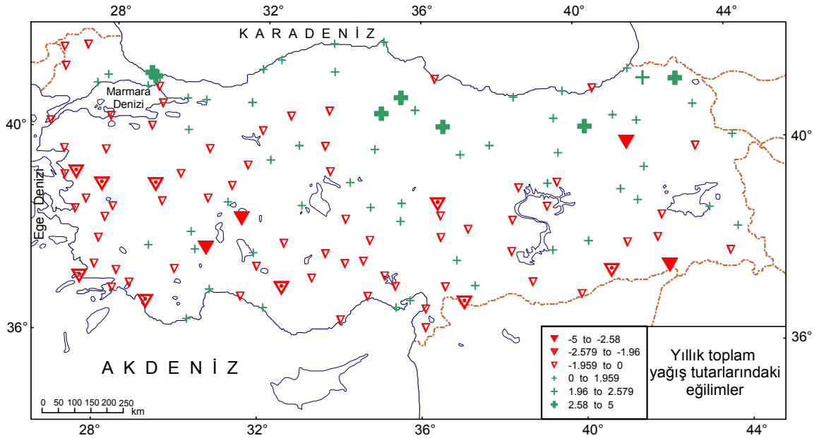
Şekil 9. M-K sıra ilişki katsayısı anlamlılık sınavına göre, Türkiye yıllık toplam yağış tutarlarındaki uzun süreli eğilimlerin alsansal dağılış desenleri. Harita açıklaması Şekil 7.1’dekinin aynıdır.
