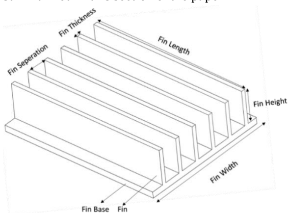
Figure 2. Geometrical fin parameters
