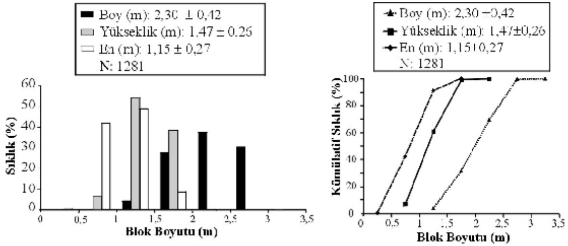
Şekil 24. Oruçoğlu Kozagaç 2 Nolu Mermer Ocağı'ndan üretilmiş olan mermer bloğu boyutlarının boy, yükseklik ve en değerlerinin, yüzde ve kümülatif dağılım grafiği
