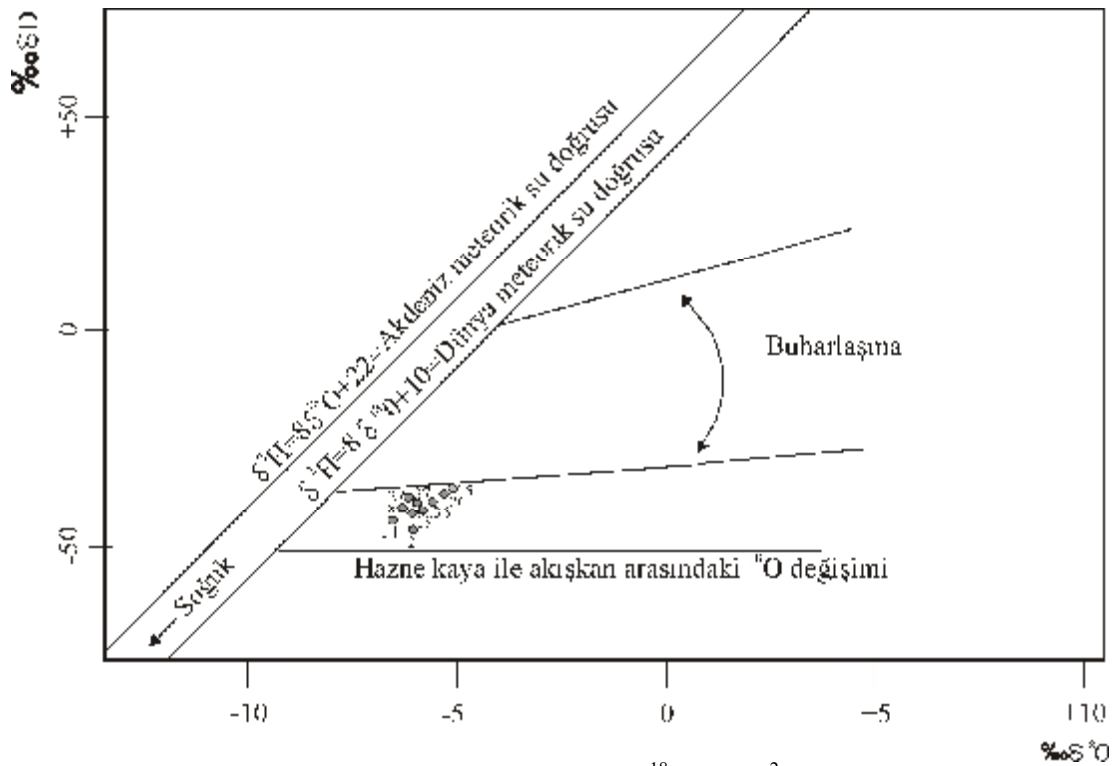
Şekil 4. Meteorik su ve doğal sularda ^{18}\text{O} ve D ( ^2\text{H} ) ilişkileri d D = 8\delta^{18}\text{O} + 22 Akdeniz meteorik su doğrusu (IAEA, 1981) d D = 8\delta^{18}\text{O} + 10 Dünya meteorik su doğrusu (Craig, 1961)
