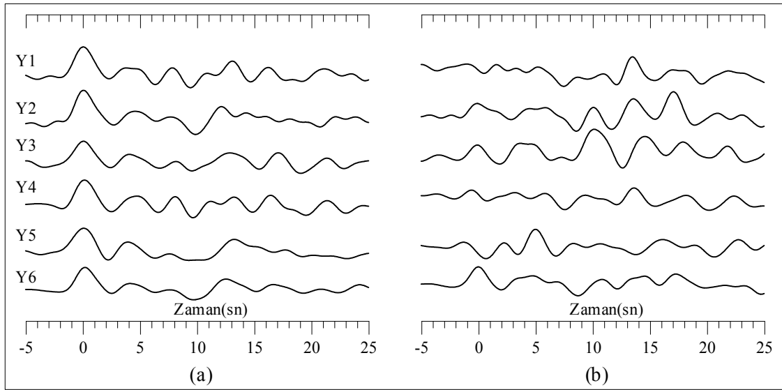
Şekil 2. Yığılma gözetimsel alıcı fonksiyonu boyuna (a) ve enine (b) dalga şekilleri
