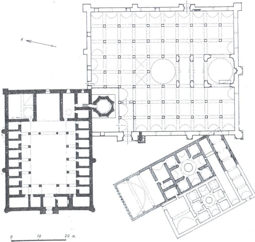
Şekil 5. Kayseri Huand Hatun Külliyesi, Plan (H. Karamağaralı, 1976)
