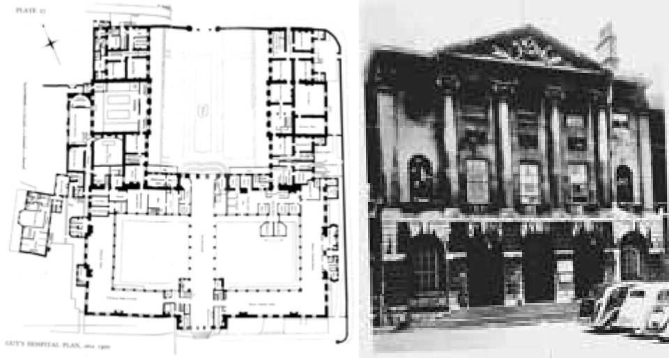
Görsel 2. Blok tip hastane örneği, Guy's Hospital plan ve görünüş, Londra.
