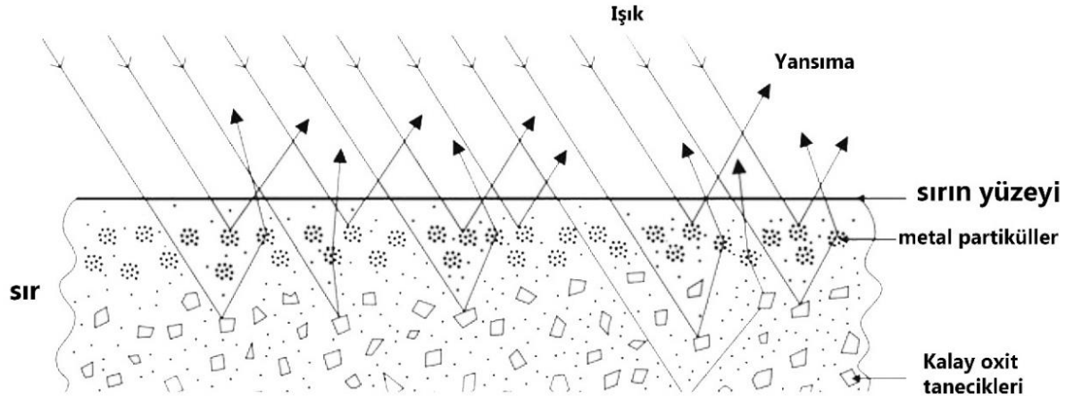
Şekil 1: Camı Bir Yüze Kismen Gömülmüş Metal Nano Partiküllerinden Oluşan Bakırmı, Altınmsı veya Yanardöner İnce Bir Film Tabakası
