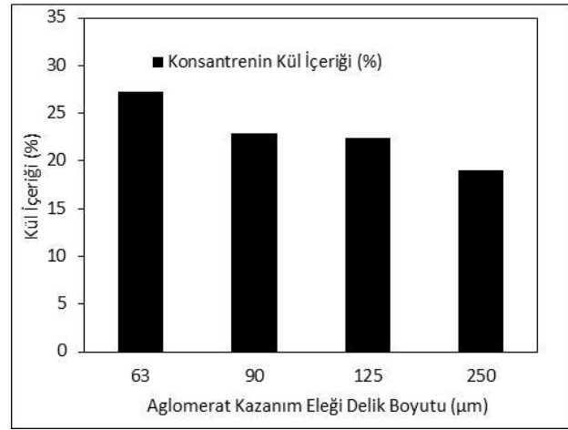
Şekil 6. Yağ aglomerasyonu deneylerinde konsantrelerin kül içerikleri.
