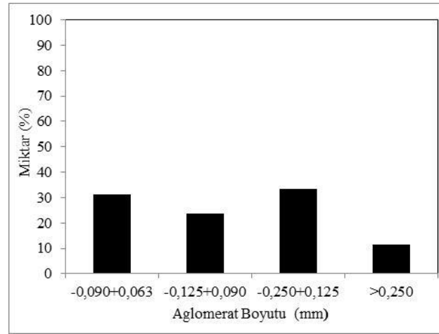
Şekil 5. Yağ aglomerasyonu deneylerinde oluşan aglomeratların boyut dağılımı.
