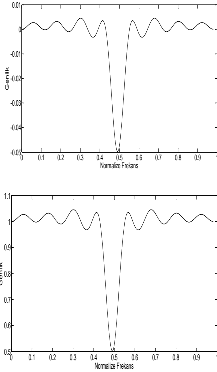
Şekil 9: N=51 için Kaiser-Hamming pencere yöntemiyle tasarlanan süzgeç bankasında. (a): Tepe yeniden elde etme hatası değişimi. (b): Genlik bozulması değişimi.
