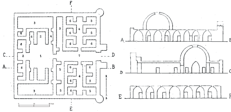
Plan 1: N. N. Pantusov tarafından çıkarılan Taş Rabat'ın ilk planı. Binanın genel planı, A-B, C-D ve E-F profillerinden görünümü (Pantusov 1916: 3-4)
