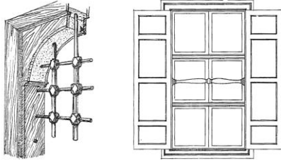
Şekil 5. Geleneksel Türk Evi'nde parmaklık ve kapaklar (Akok, 1957)
