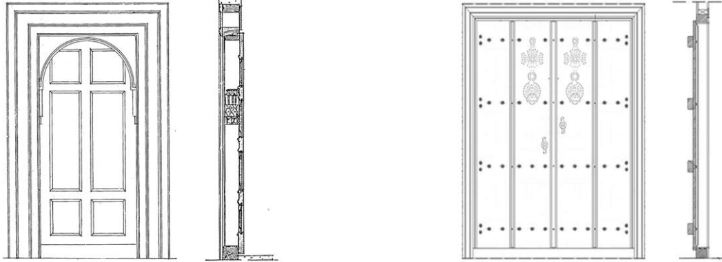
Şekil 2. Oda kapısı detayları (Akok, 1995)
