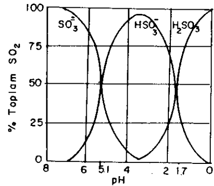
Şekil 2. Kükürt dioksit üzerine pH'nın etkisi (25°C)
