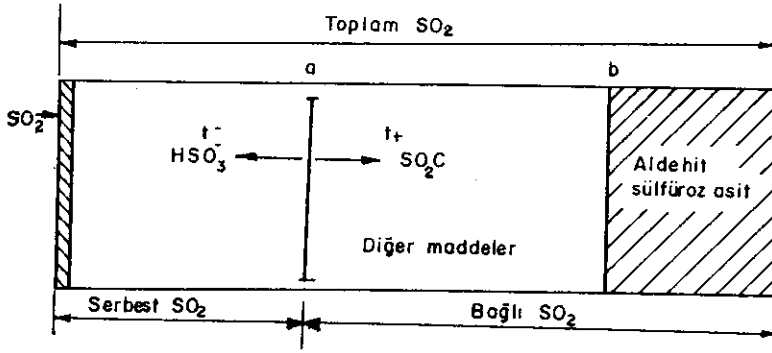
Şekil 1. Şarapta kükürt dioksitin değişik durumları.
