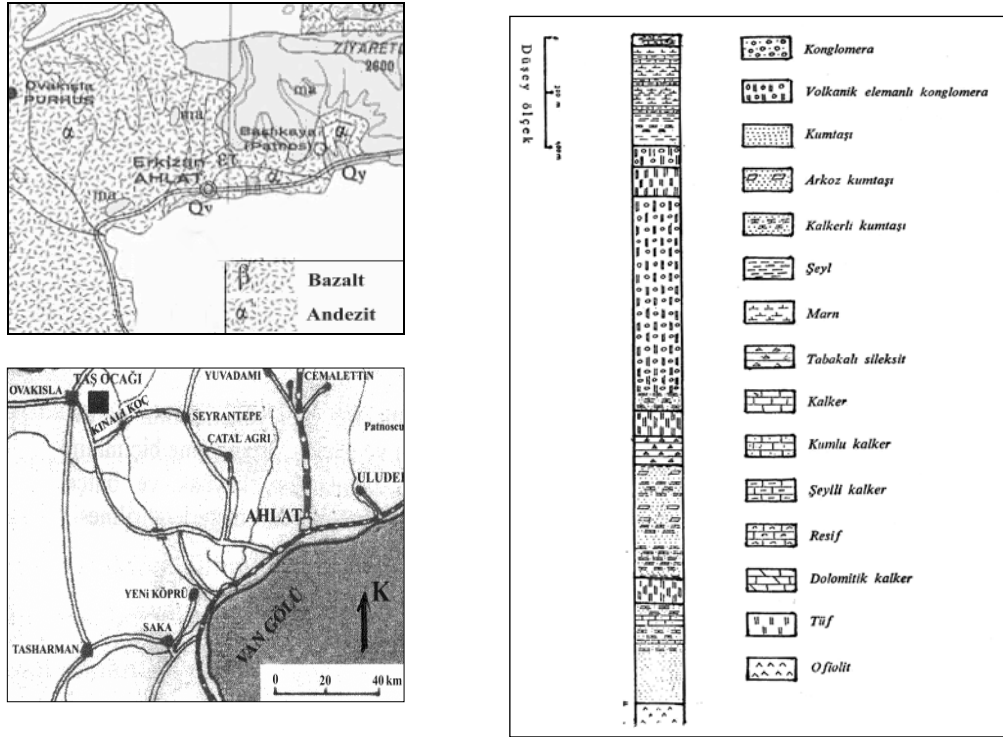
Figure 2. The geological map and the stratigraphical section of the rock quarry Şekil 2. Taş ocağının jeolojik haritası, mevki haritası ve dikme kesiti
