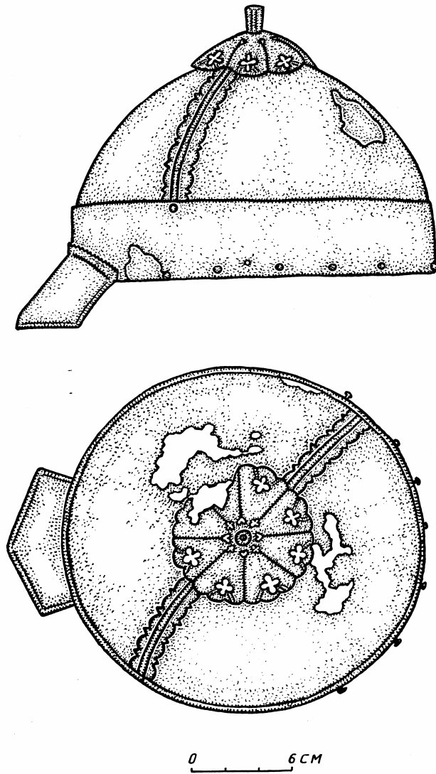
Рис. П. Шлем из Ак-Келя: 1 - вид спереди, 2 - вид сзади.
