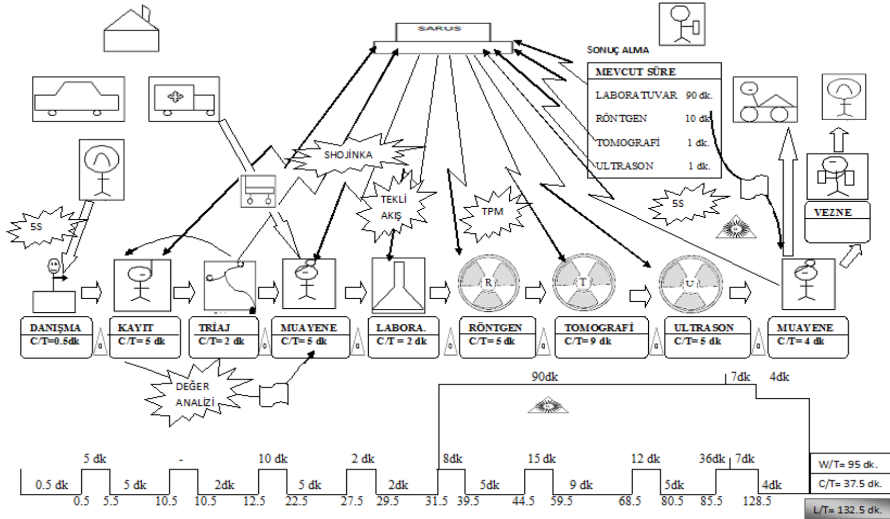
Şekil 4. Kaizen Noktalı Mevcut Durum Haritası
