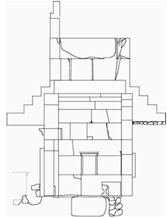
Fig. 14. Hellenistik Anıt Mezar Kesit Görünüşü
