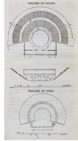
Fig. 3. Patara ve Myra Tiyatroları Cavea ve Sahne Binası Planı ve Restitüsyonu
