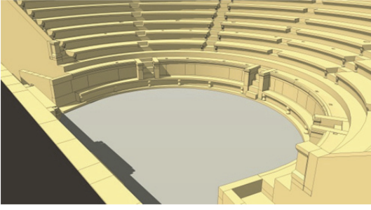
Fig. 39b. Rhodiapolis Tiyatrosu Cavea Rekonstrüksiyonu
