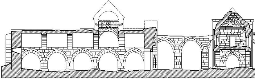
Afyon-İshaklı Sâhip Ata Kervansarayı ana Kesiti (Hicazî Kesit İstikametine Çizilmiştir) (V.G.M. Abd. Yp. İş.Dai. Bşk.Arşivi'nden Düzeltildi)
