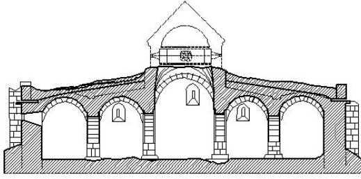
Afyon-İshaklı Sâhip Ata Kervansarayı Kesiti (E.İ.İ. Abd. Yp. İş.Dai. Bşk.Arşivi'nden Düzeltildi)
