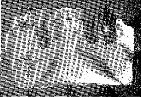
Resim 6: İzokromatik çizgilerin görünümü
