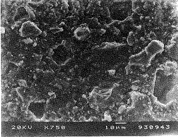
Resim 1.C- 60 sn. asit uygulanmış düz yüzey
