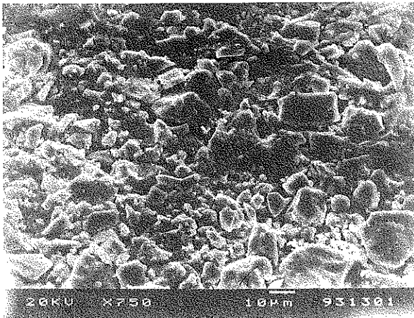
Resim 1.D- Normal açık havada sertleştirilmiş, asit uygulanmamış yüzey
