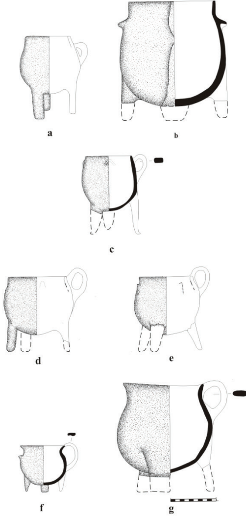
Levha 10: a-b: B2 Tipi , a: Thermi, İTÇ II (Lamb, Exavations at Thermi in Lesbos, s. 125: plt.IX-440), b: Kusura, İTÇ II (Lamb, "Excavations at Kusura Near Afyon Karahisa", s. 19-21: fig.7-2), c: B3 Tipi Küllüoba, İTÇ II (Efe "Two Burnt Rooms at Küllüoba Near Eskişehir", s. 116-127:17), d-g: C1 Tipi, d-e: Thermi, İTÇ I (Lamb Excavations at Thermi in Lesbos, s. 100: plt.XXXV-27; 114: plt.XXXVI-258), f: Beyesultan, İTÇ I (Lloyd ve Mellaart Beyesultan Vol.I , s. 123: fig. 16/16), g: Bademağacı, İTÇ II (Duru ve Umurtak "Bademağacı Kazıları 2000", ss. 240-244 res.3, Duru "Bademağacı Kazıları 2000 ve 2001", Lev.31.3 Lev.42.4, Türkiye'deki (Üstün), "Bademağacı İlk Tunç Çağı II Kırmızı Astarlı Mallar" Lev.47.1).
