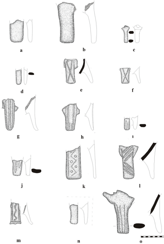
Levha 13: a-o: A Tipi, a: Kumtepe, İTÇ'ye Geçiş (Sperling a.g.m., s. 337: fig. 18.558), b: Kahlık Mevkii, İTÇ'ye Geçiş (Efe, İlaşlı ve Topbaş a.g.m., s. 385: fig.24.80), c-d: Aphrodisias, İTÇ II (Joukowsky a.g.e., ss. 544-546: Lev.392.27; ss.582-583: Lev.421.33), e: Manclarlı, İTÇ II (Mellaart "Survey of Pre-Classical Remains in Southern Turkey", çiz.212), f: Karataş-Semayük, İTÇ II (Eslick a.g.e., ss. 203-204: KT233), g: Beycesultan, İTÇ II (Lloyd ve Mellaart Beycesultan Vö.I. s.189: fig.46.11), h: Karataş-Semayük, İTÇ II (Eslick a.g.e., s.158. KT530), i-j: Aphrodisias, İTÇ II (Joukow a.g.e. s. 580-583: Lev.421.27; 579-583: Lev.421.34), k-l: Beycesultan, İTÇ II (Lloyd ve Mellaart Beycesultan Vö.I. s.151: fig.26.9; 189:fig.46.12), m: Manclarlı, İTÇ II (Mellaart "Survey of Pre-Classical Remains in Southern Turkey" çiz.213), n: Bademağacı, İTÇ II (Türkteki (Üstün) "Göller Bölgesi İlk Tunç Çağı 1-2 Çanak Çömleği", Lev.52.4), o: Aphrodisias, İTÇ IIIa (Joukowsky a.g.e., ss. 640-642: Lev.462.11).
