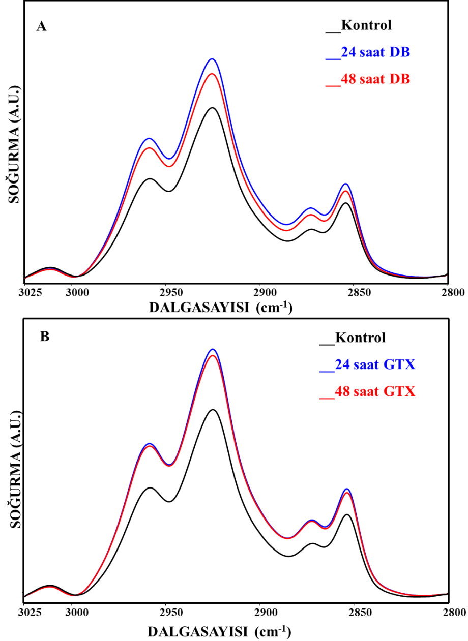
Şekil 3. Kontrol, DB (A) ve GTX (B) uygulamasından 24 ve 48 saat sonra incelenmiş fare karaciğer dokularının 3025-2800 \text{cm}^{-1} dalga sayısı aralığındaki spektrumları (Spektrumlar Amid A bantına göre normalize edilmiştir).
