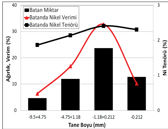
Şekil 9. Ağır sıvı test sonuçları (Batan Ürünler)
