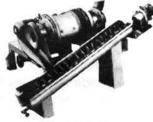
BİLYALI ÇUBUK DEĞ.
