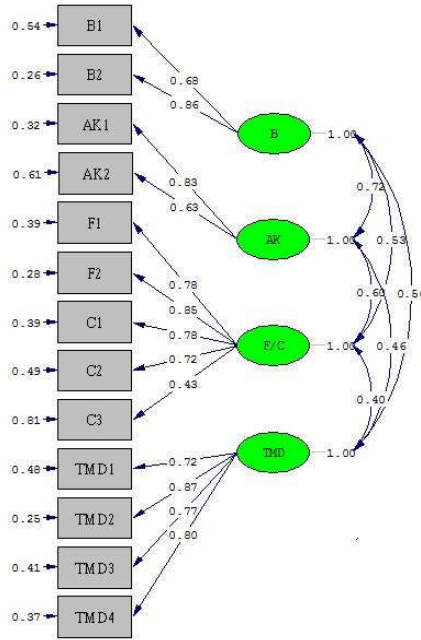
Şekil 3. Doğrulayıcı Faktör Analizi
