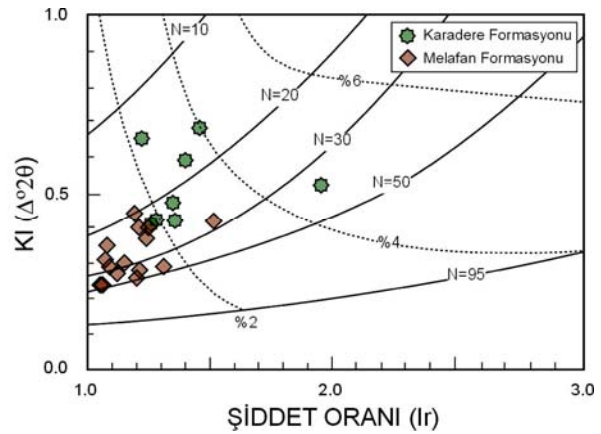
Şekil 6. Maden Grubu illitlerinin kristalinite ve şiddet oranı diyagramına (Eberl ve Velde, 1989) göre kristalit büyüklüğü ve % smektit içerikleri.
