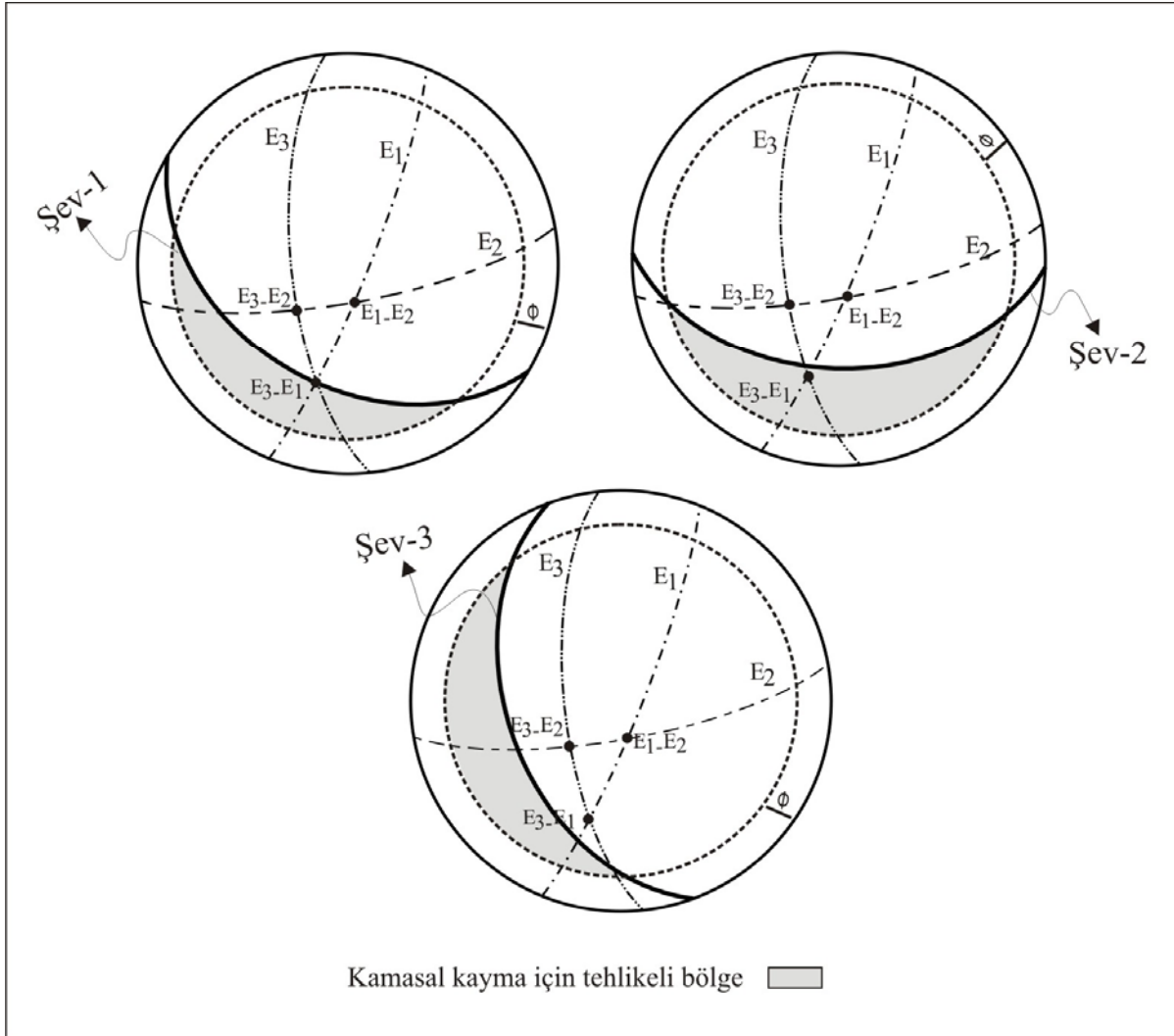
Şekil 12. Bayhasan-Kızık civarındaki kaya şevlerinin duraylılığının kinematik analizi.
