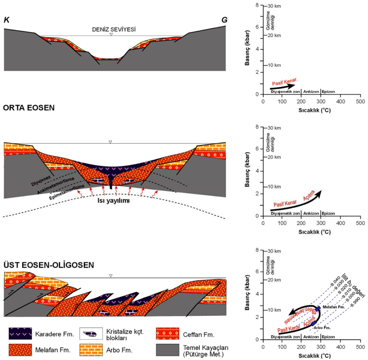
Şekil 14. Maden Grubu'nun açılmalı basen ortamında sıcaklık-basınç-zaman (P-T-t) tersi yöneliminin şematik gösterimi.
