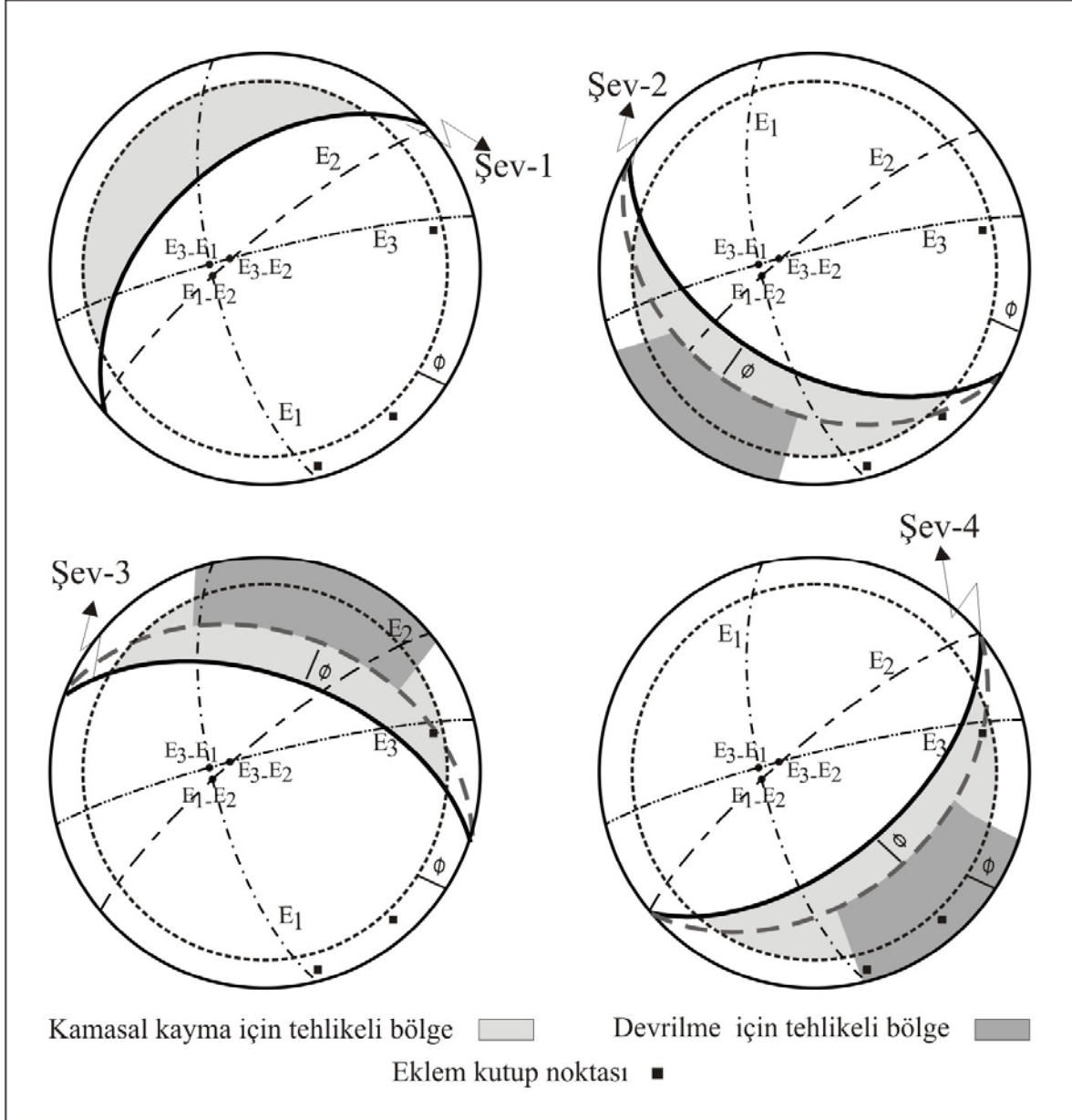
Őekil 14. Kale tepe civarındaki kaya Őevlerinin duraylılıđının kinematik analizi.
