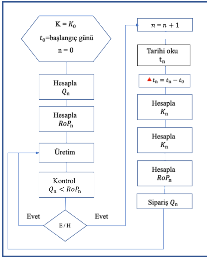
Şekil 5:Önerilen Dinamik QR Algoritması
