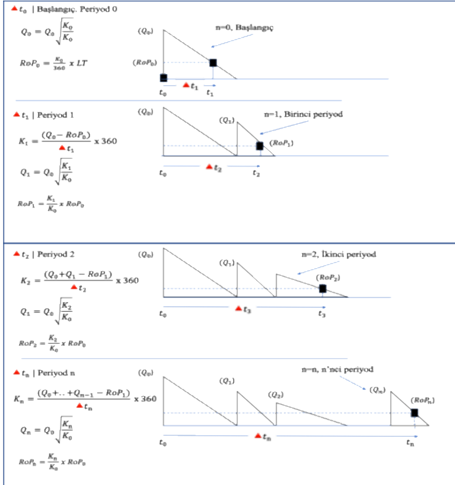
Şekil 8: Algoritma Formülleri
