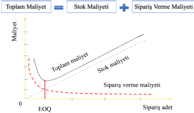
Şekil 4: Ekonomik Sipariş Miktarı (EOQ)
