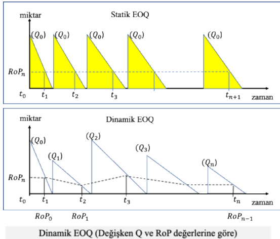
Şekil 6: Algoritmanın Simülasyonu
