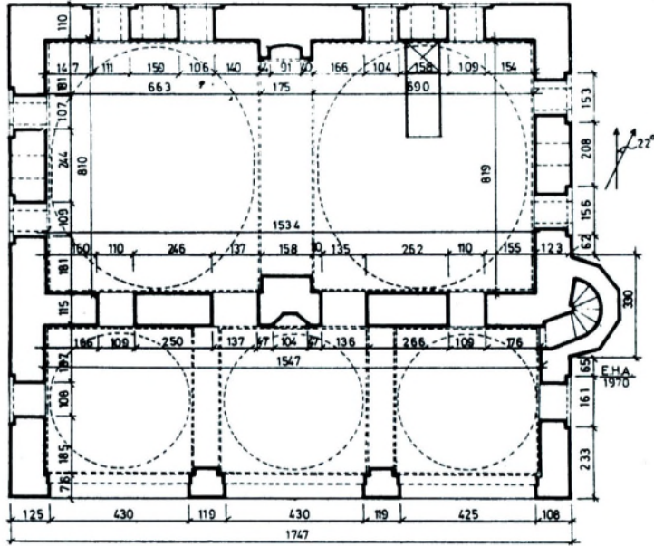
Şekil 9 - Bursa Abdal Mehmed Camii planı (E.H. Ayverdi'den)
