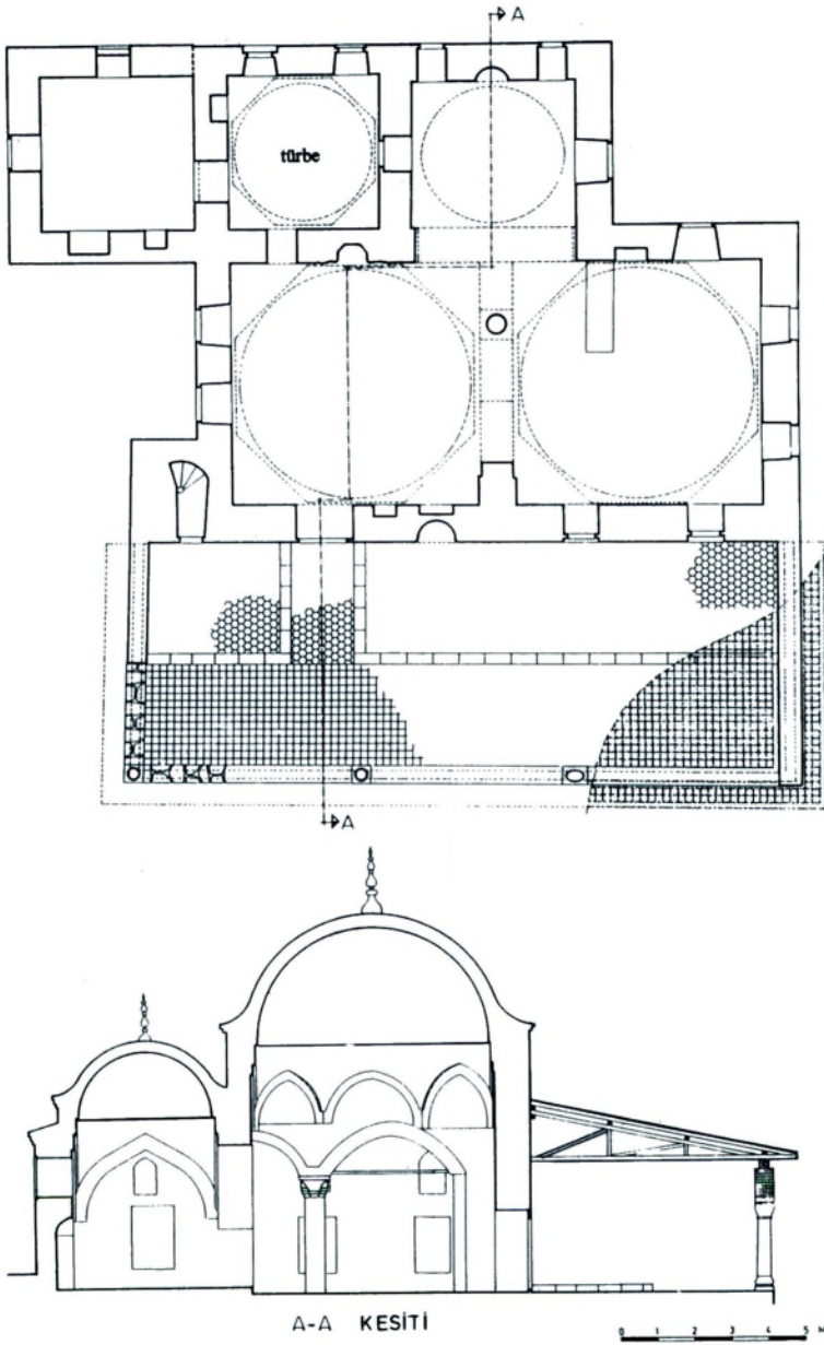
Şekil 1 - İskilip Şeyh Yavsi Camii plan ve kesiti (A. Kılıcı'dan)
