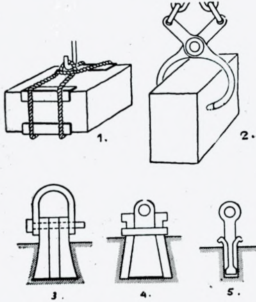
Res. 12 — Kaldırma şekilleri (Binan'dan): 1 — Bağlayarak, 2 — Kanca bacak ismi verilen bir nevi kısaç, 3-4 — Kumtaşları için kurt ağzı, 5 — Granit taşlar için kurt ağzı.
