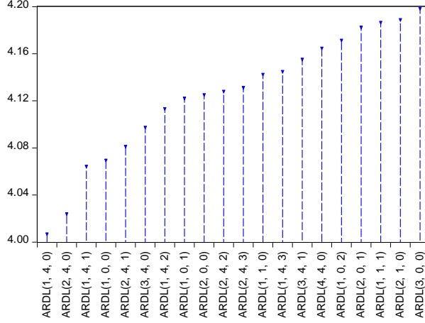
Grafik 4. Uygun Gecikme Uzunluğunun belirlenmesi (model) Akaike Information Criteria (top 20 models)
